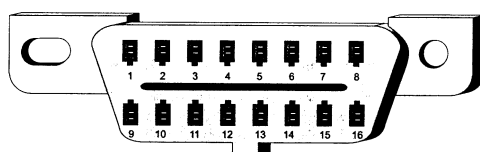
Interface de connexion OBD
