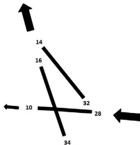
Skizze 3: Ostanflugkonzept
